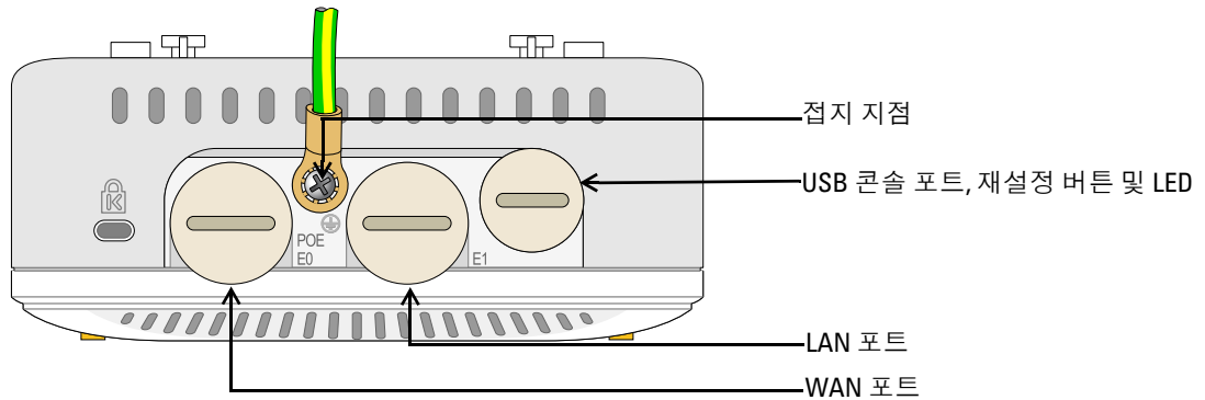
그림 2 W-AP228 하단 보기
