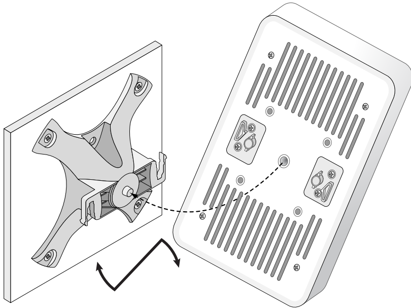
그림 7 장착 브래킷에 AP 부착
